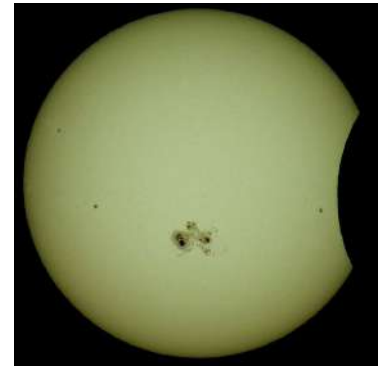
Above: sunspots. Below: Sun surface. / Boven: Zonnevlek. Beneden: Zon oppervlakte
