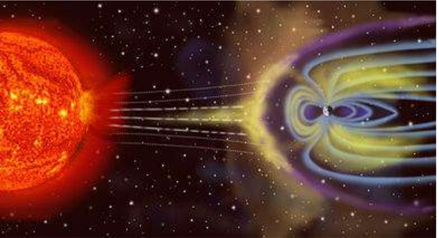
Above: The earth has its own magnetic field. / Boven: De aarde heeft haar eigen magnetische veld.
