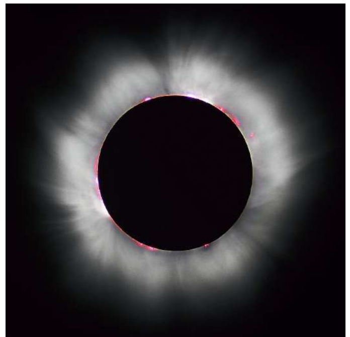
Above: sun. Right: solar eclipse with corona visible. / Boven: Zon. Rechts: Zonsverduistering met corona zichtbaar.
